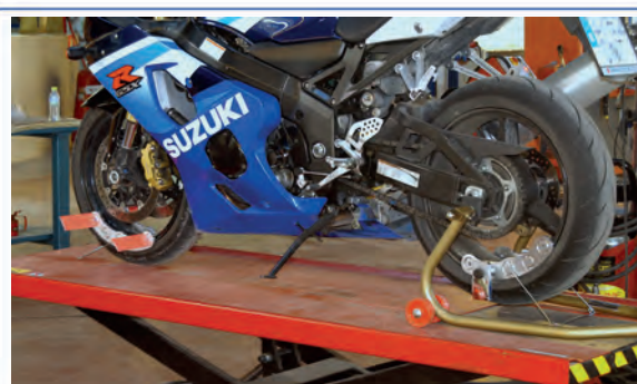
8 Medición del paralelismo o alineación, entre la rueda delantera y la trasera.
